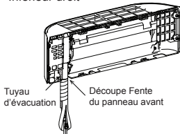
Tuyau d'évacuation
